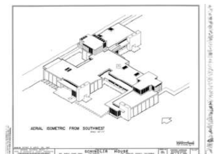
Rudolph SCHINDLER, Schindler house , 1922, vue axonométrique.
