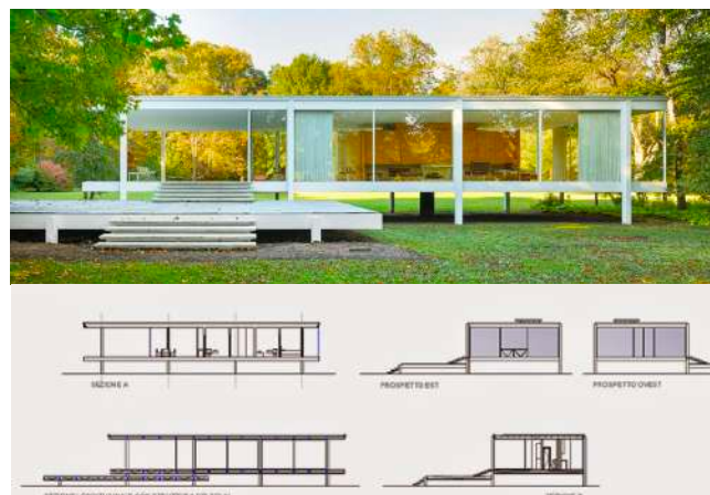
Mies van der Rohe, Farnsworth house, 1945-51.
